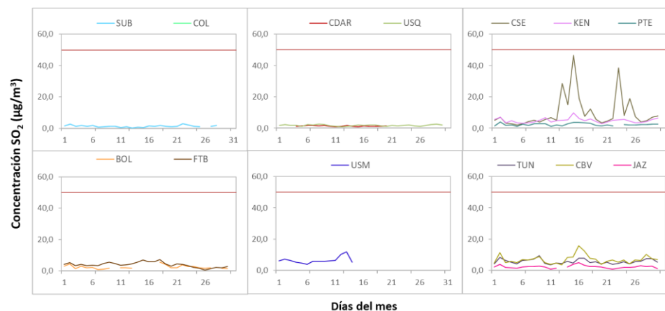
Figura 14. Concentraciones promedio mensuales de SO_2 por estación de monitoreo - junio 2022
