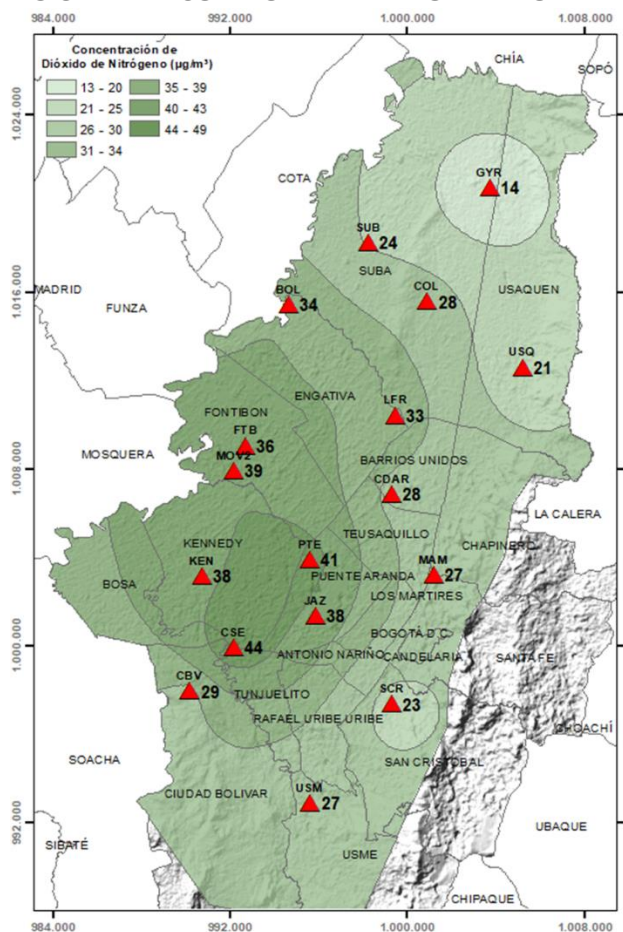
Figura 15. Distribución espacial concentraciones mensuales NO 2 - junio 2022
