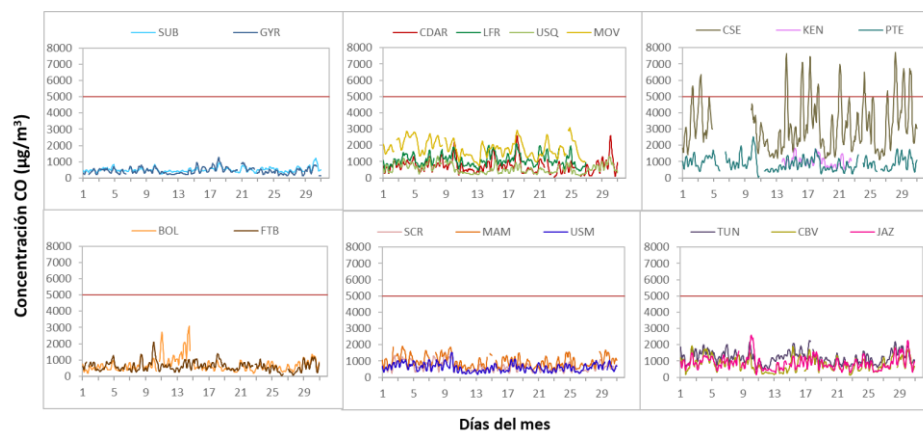
Figura 18. Concentraciones media móvil 8 horas de CO por estación de monitoreo - junio 2022
