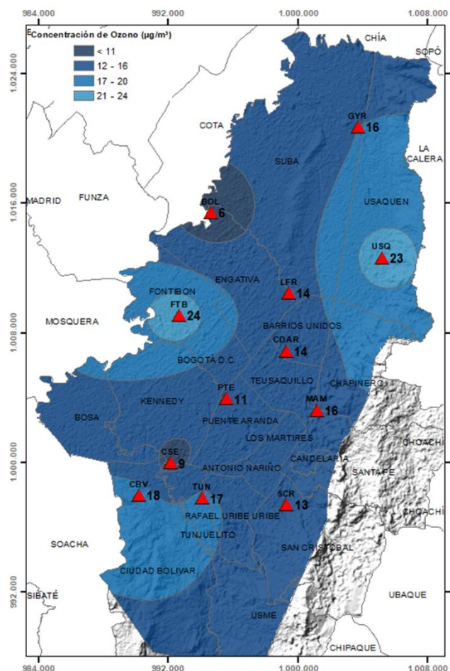
Figura 10. Distribución espacial concentraciones mensuales O 3 – junio 2022
