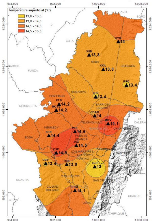
Figura 29. Mapa del promedio de temperatura superficial de las estaciones de la RMCAB con base en el método de interpolación de Kriging – junio 2022
