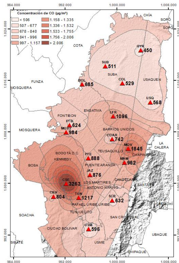
Figura 17. Distribución espacial concentraciones mensuales CO – junio 2022
