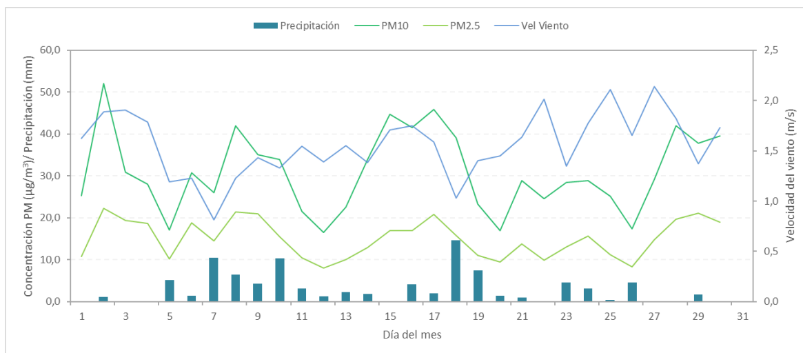
Figura 6. Promedio de concentración PM 10 y PM 2.5 , precipitación y velocidad del viento a nivel ciudad – junio 2022
