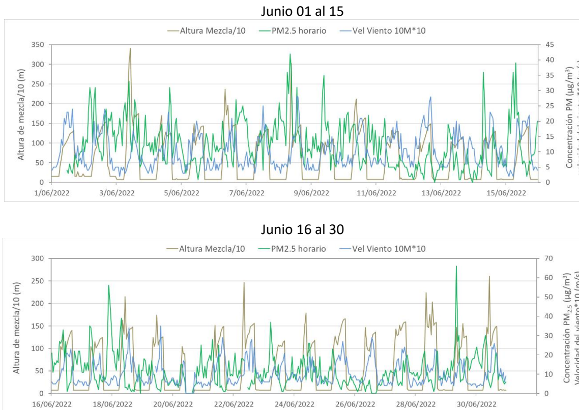
Figura 8. Comparación altura de mezcla, concentraciones PM_{2.5} y velocidad del viento estación Guaymaral - junio 2022
