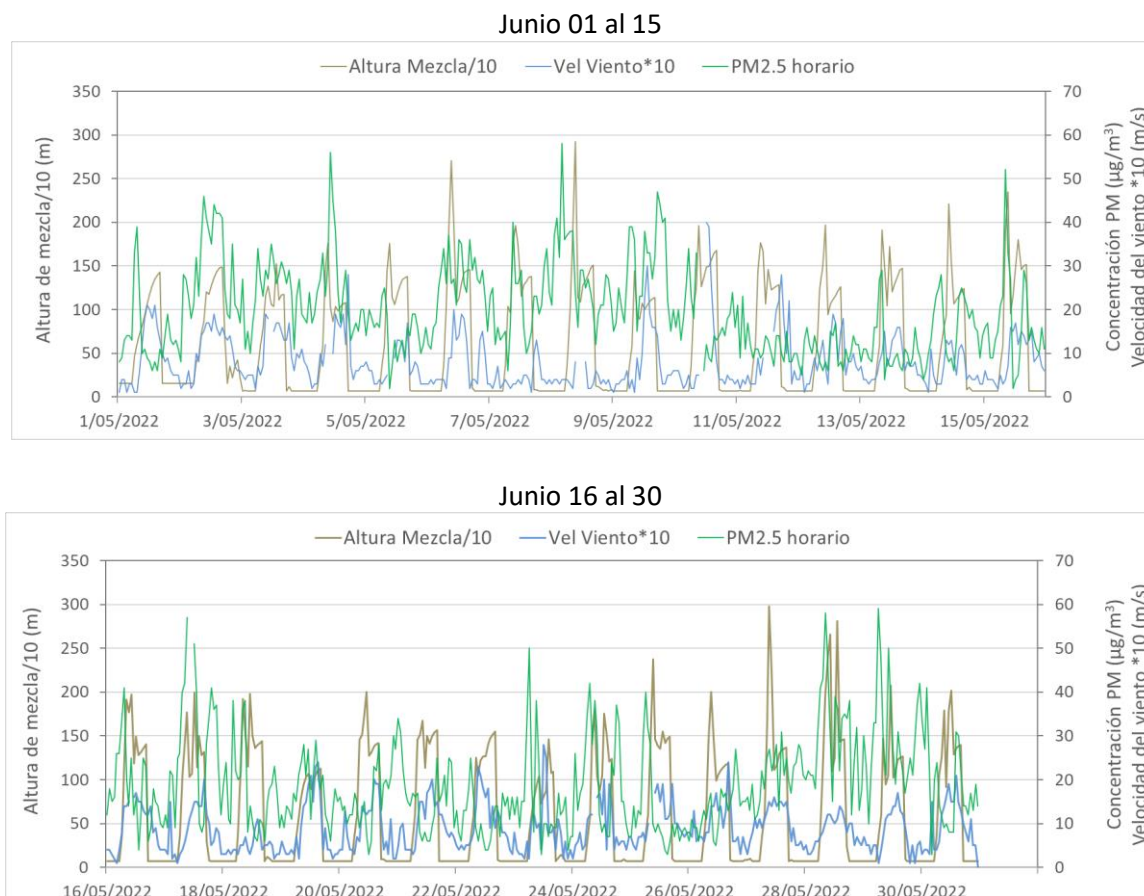
Figura 7. Comparación altura de mezcla, concentraciones PM 2.5 y velocidad del viento estación Tunal - junio 2022
