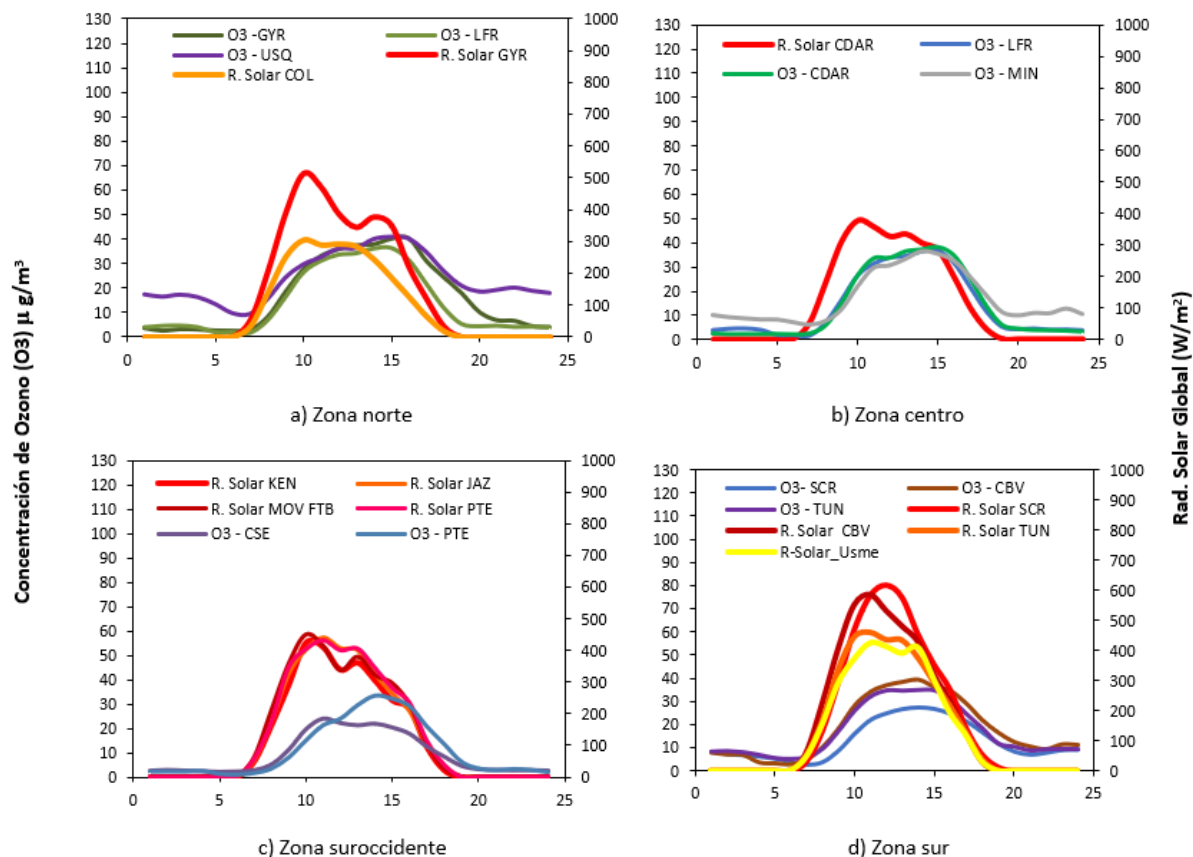
Figura 12. Comportamiento horario de las concentraciones de O_3 ( \mu g/m^3 ) y su relación con la Radiación Solar entrante ( W/m^2 ) – junio 2022. a) zona norte, b) zona centro, c) zona suroccidente y d) zona sur
