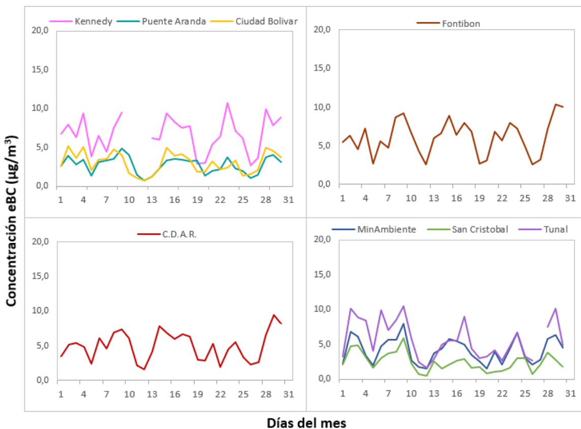
Figura 19. Comportamiento de las concentraciones diarias de BCE para junio 2022
