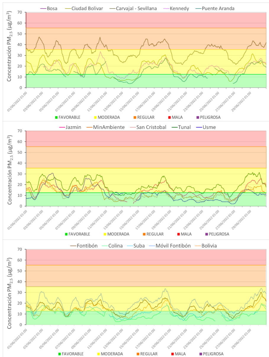
Figura 26. Concentraciones media móvil 24 h PM 2.5 junio 2022
