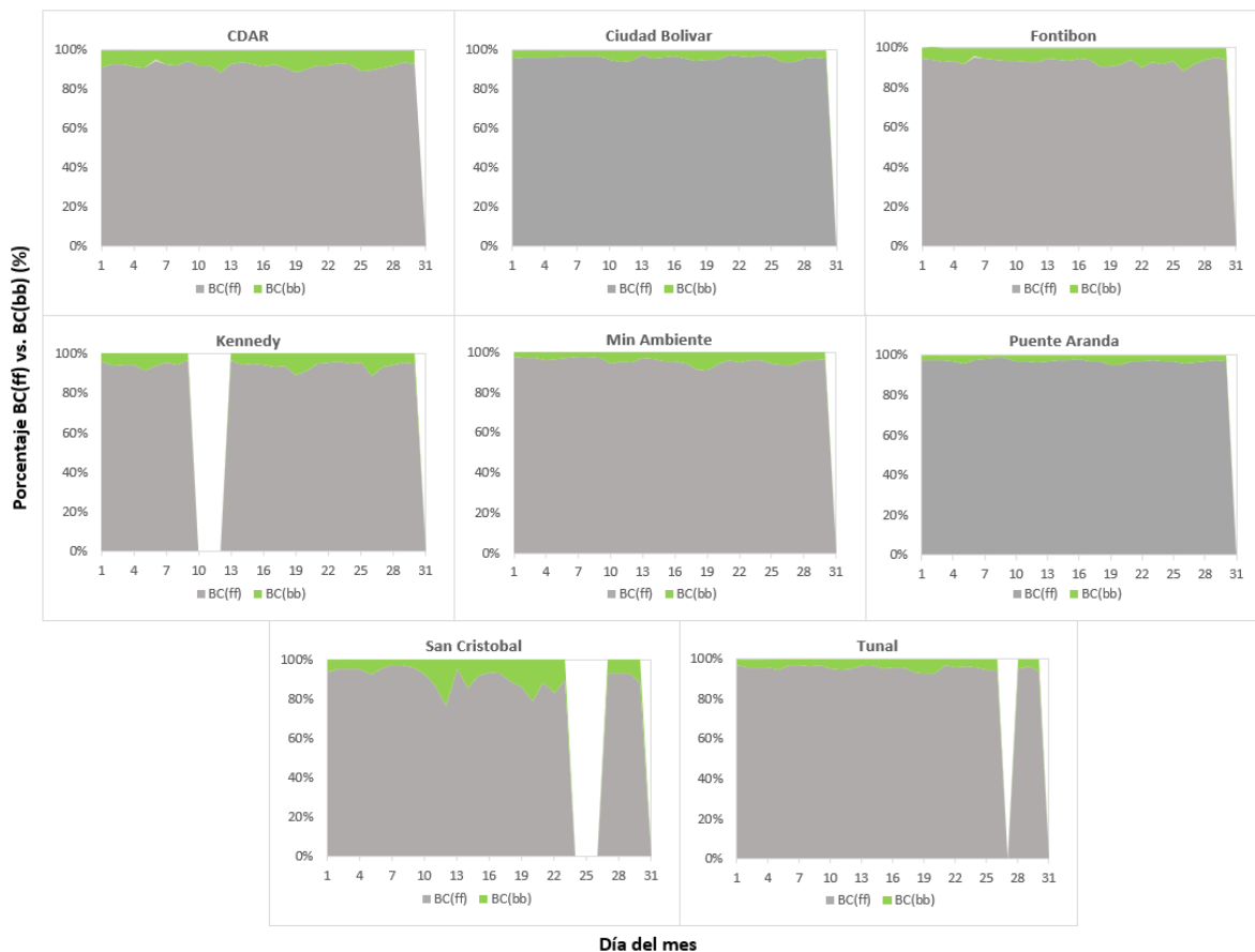
Figura 22. Serie temporal porcentaje de quema Black Carbon de combustibles fósiles BC(ff) vs. Black Carbon de quema de biomasa BC(bb) – junio 2022
