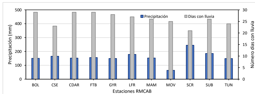
Figura 28. Precipitación media mensual y número de días con precipitación – junio 2022
