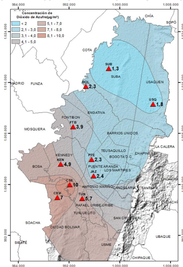
Figura 13. Distribución espacial concentraciones mensuales SO_2 – junio 2022
