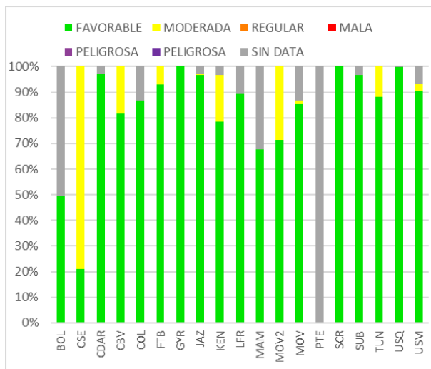
Figura 23. IBOCA para PM 10 por estación – junio 2022
