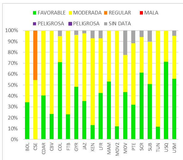
Figura 24. IBOCA para PM 2.5 por estación – junio 2022
