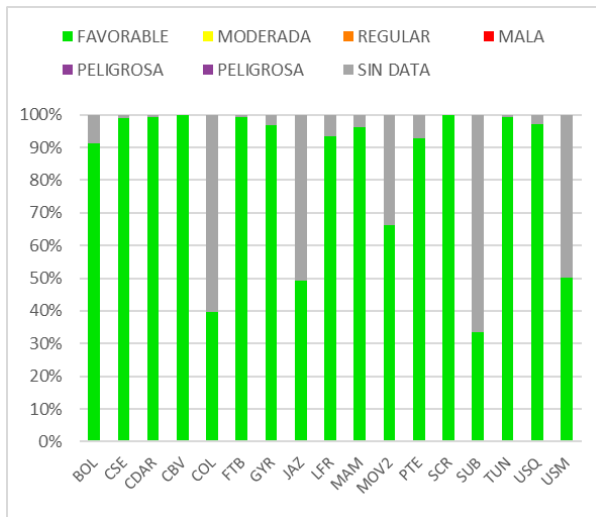
Figura 25. IBOCA para O 3 por estación – junio 2022
