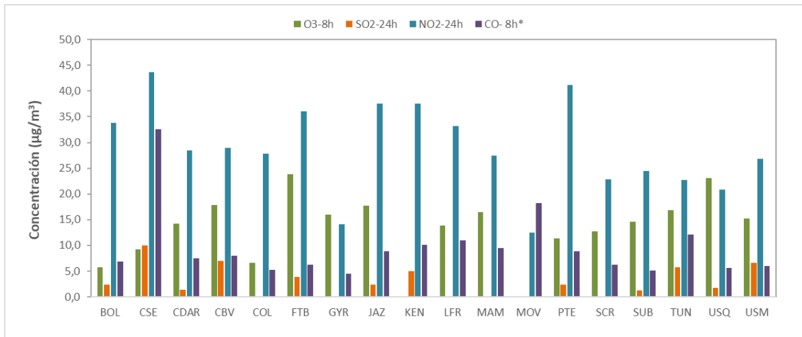
Figura 9. Concentraciones mensuales de gases (O 3 , SO 2 , NO 2 y CO) por estación de monitoreo - junio 2022
