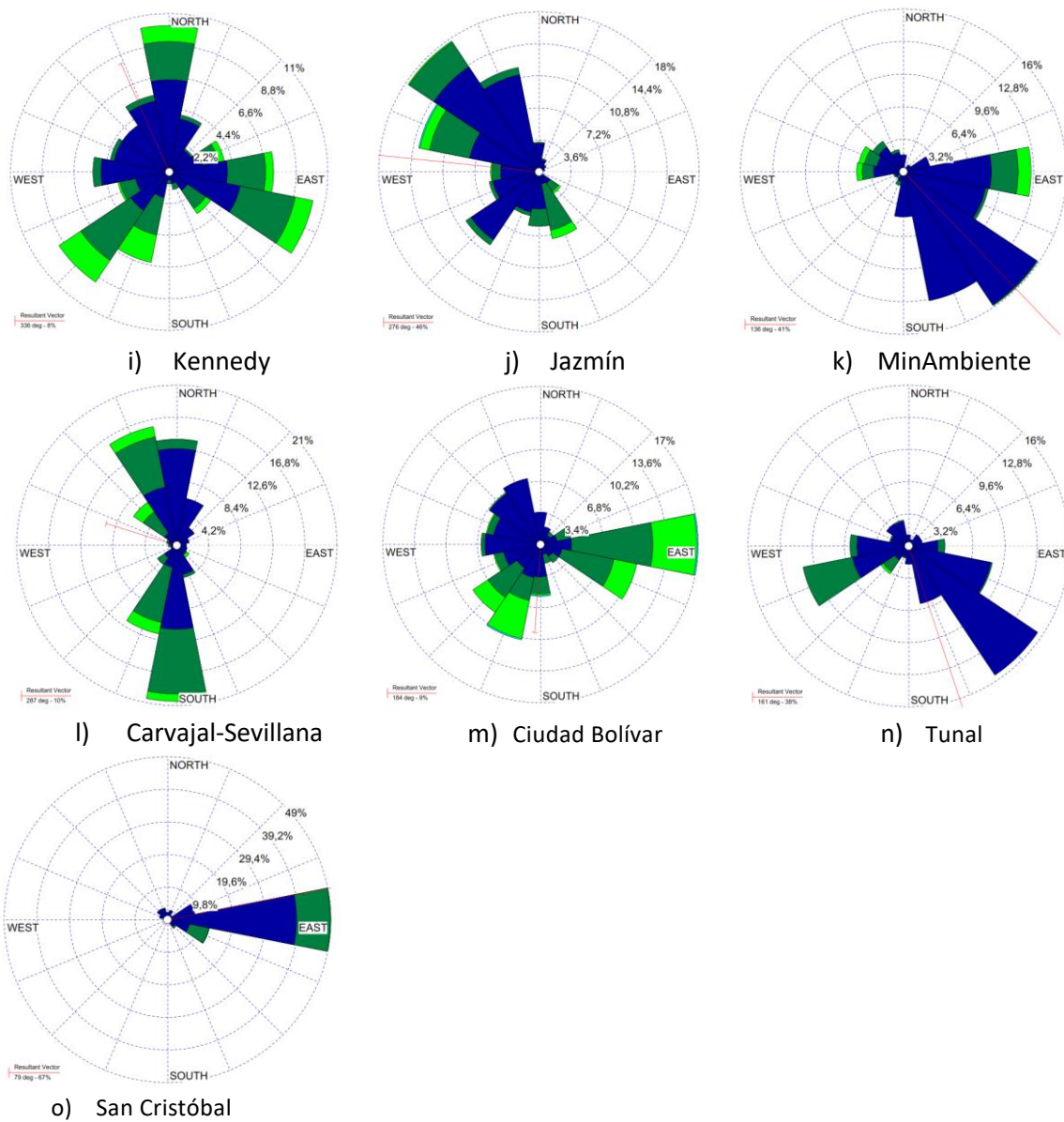
Figura 33. Rosas de los vientos – junio de 2022
