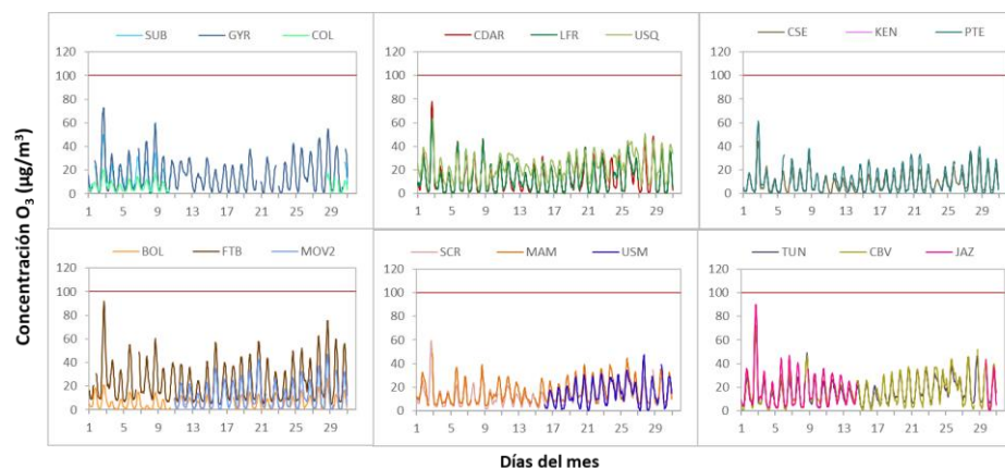
Figura 11. Concentraciones media móvil 8 horas de O 3 por estación de monitoreo - junio 2022
