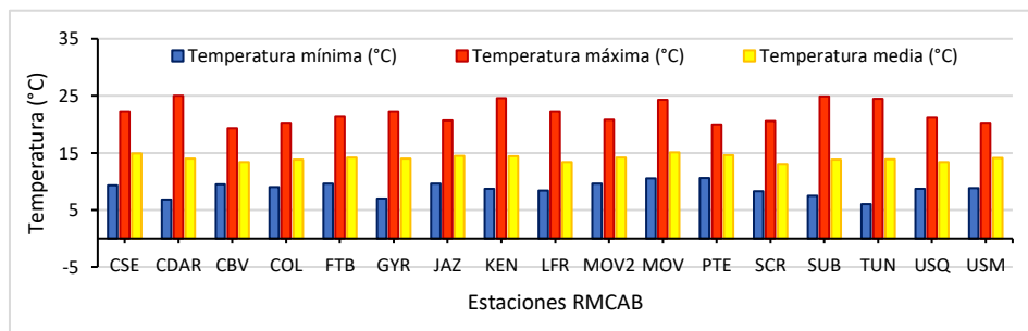
Figura 30. Temperaturas medias, máximas y mínimas absolutas por estación – junio 2022
